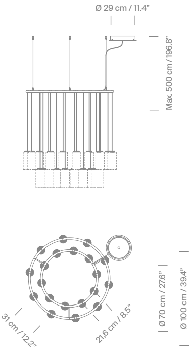
Example direct cable to ceiling / Ejemplo cable directo a techo
